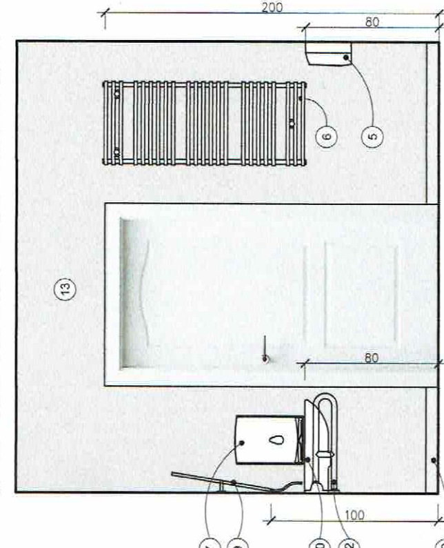
Widok D-A
