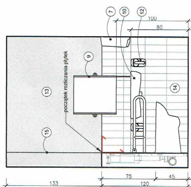
Widok C-D
